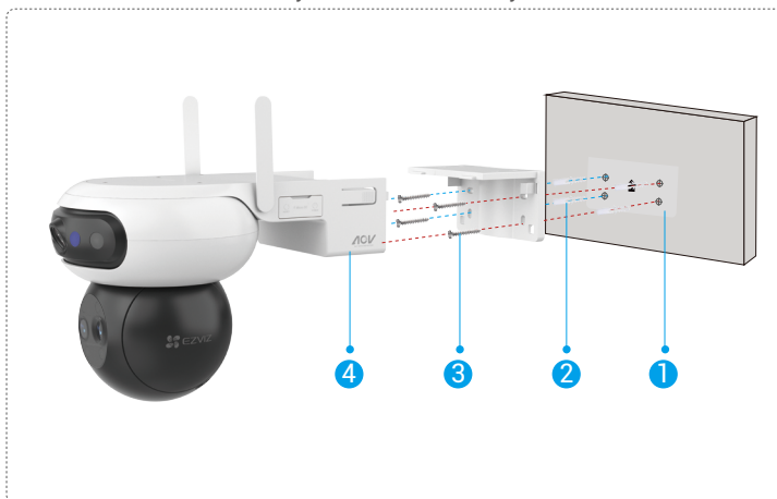
Rys. 2 Montaż ścienny
